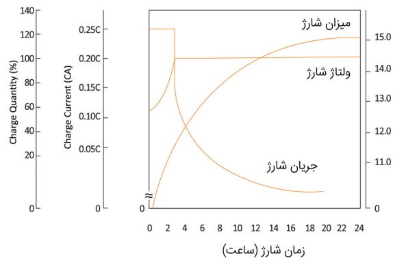
منحنی مشخصه شارژ ( 25^{\circ}\text{C} )
